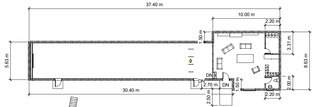
1 Level 0 1 : 200
