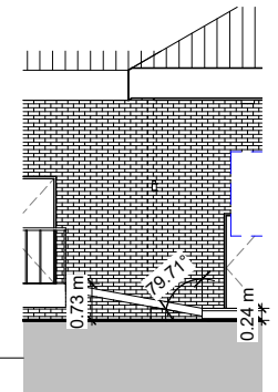
4 Section 3 1 : 100
