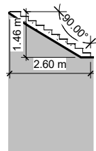
2 Section 1 1 : 100
